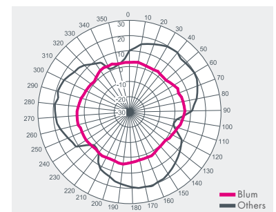
Повышенная точность за счет круглого измерительного механизма
